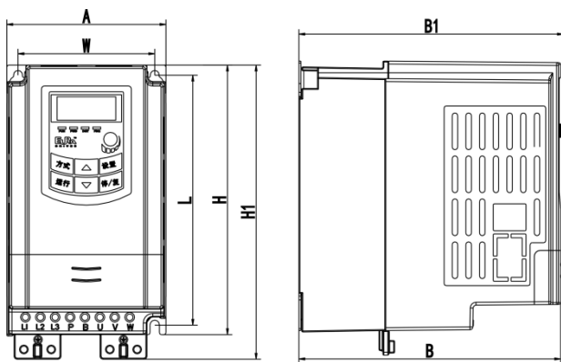
塑壳外形
