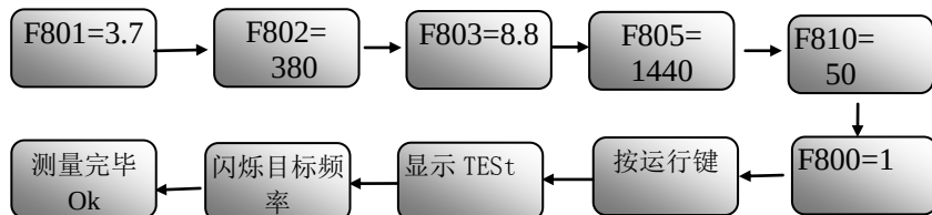
图 6-22 参数测量流程图
