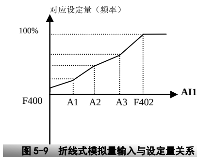
图 5-9 折线式模拟量输入与设定量关系
