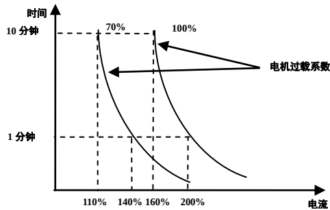
图 5-12 电机过载系数设定
