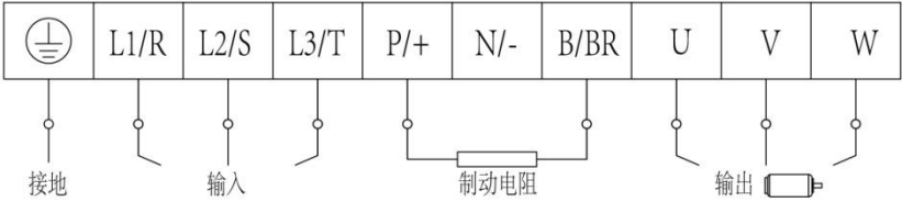
图 3-4 端子示意图
