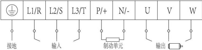
图 3-6 端子示意图
