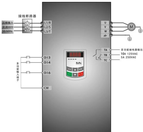
图 4-2 接线图 2
