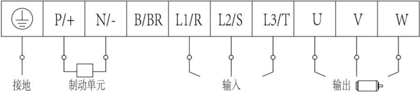
图 3-5 端子示意图
