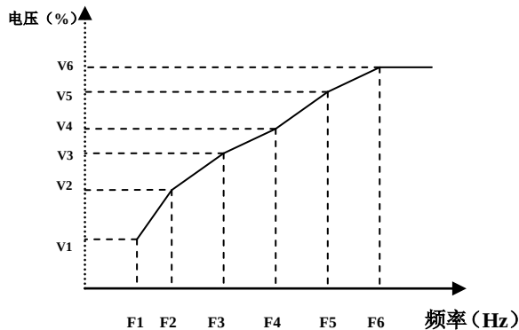
图 5-4 VVVF 曲线设定示意图
