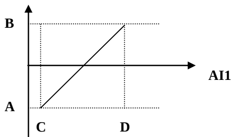
图 5-8 模拟给定与设定量的计算关系
