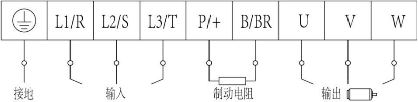
图 3-3 端子示意图
